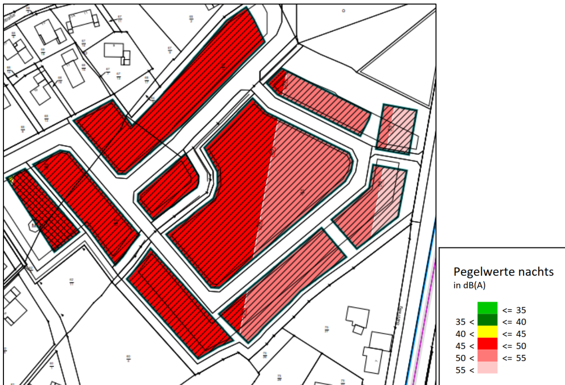
Abbildung 5: Rasterlärnkarte für die Vorbelastung Verkehrslärm (Schiene) nachts im OG
