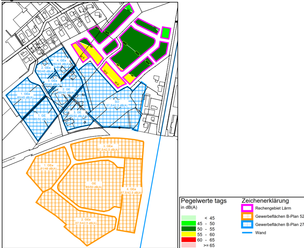
Abbildung 6: Rasterlärkarte für die Vorbelastung Gewerbelärm tagsüber
